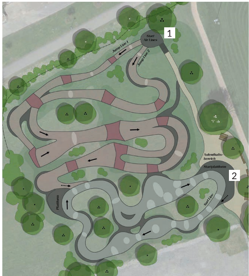
Projektskizze der Pumptrackanlage auf einer Teilfläche der Rüeggiswilwiese: (1) Der Start zu den Air Lines (Jump Line 1 und 2) (2) Die Startplattform der Surf Line.
