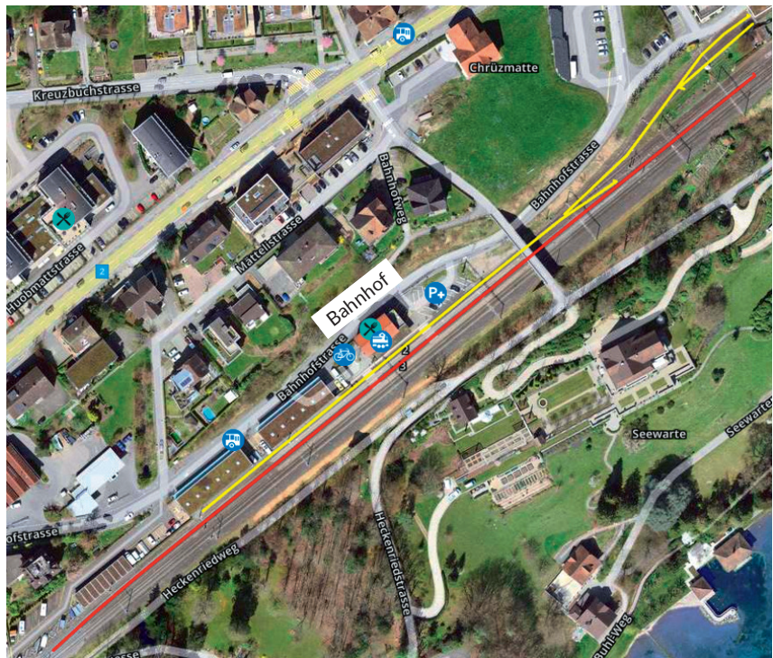
Abschnitt Gleisbauarbeiten im Bahnhof Meggen: Rot Umbau, gelb Abbruch.
