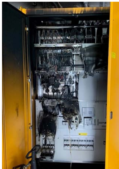
6. Juli 2023: Die elektrische Hauptverteilung nach dem Brand.
