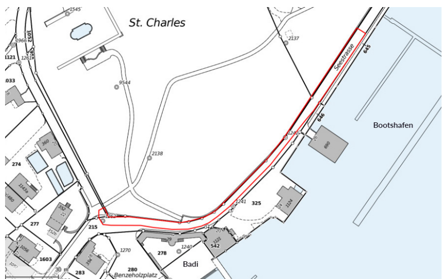
Situation Baubereich Sanierung Wasserleitung im Abschnitt Benzeholzplatz bis Bootshafen an der Seestrasse.
