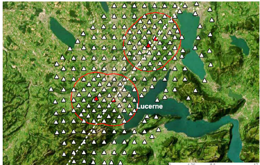
Standorte der geophysikalischen Untersuchungen des Untergrundes.
